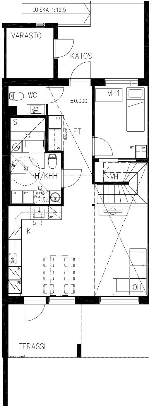
1. KERROS
